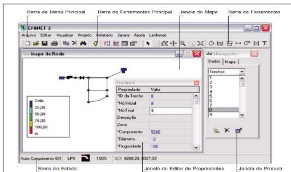
Figura 7: Configuração básica do ambiente de trabalho do EPANET
