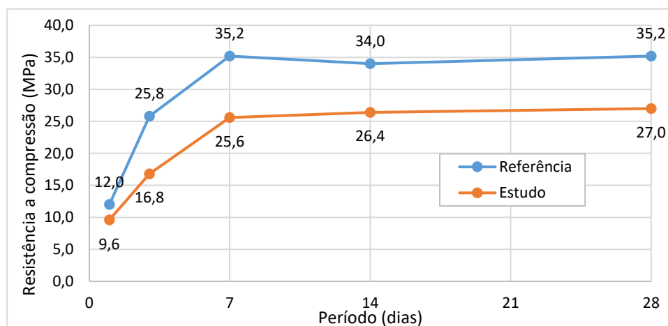
Figura 6 – Resultado do ensaio de resistência à compressão ao longo dos dias para os corpos de prova referência e de estudo.
