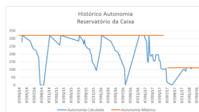
Figura 43: Análise histórica da Autonomia - Reservatório Rio da Caixa - SAA Rio do Pires
