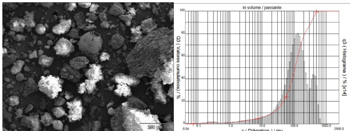
Figura 5 – Micrografia da cinza com 2 h de moagem
