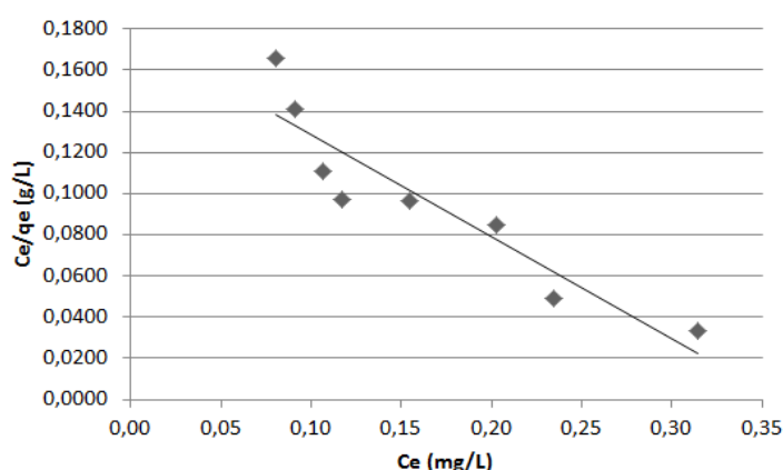
Figura 91. Isotherma de Langmuir para a adsorção do AM pela argila bentonita.
