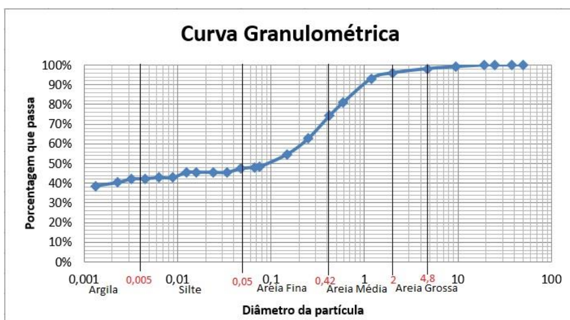
Figura 3: Curva granulométrica do Solo
